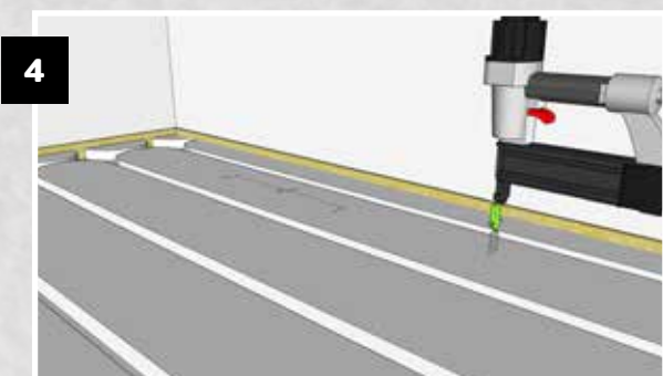
Niet het element vast met spreidnieten 35-40mm h.o.h. 200mm
