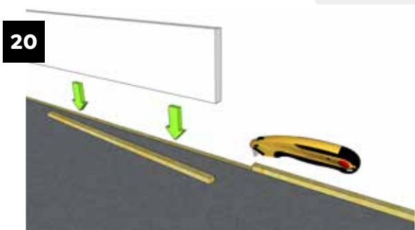
Kantstroken wegsnijden en plinten plaatsen
