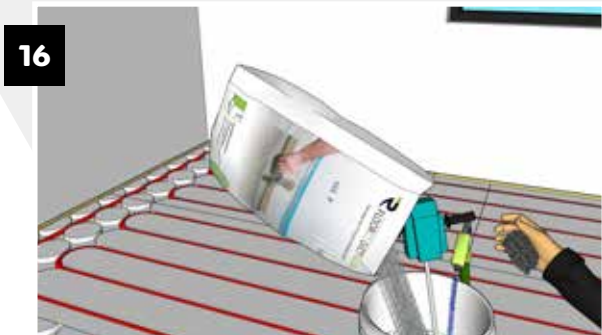
16 Gietmassa mixen met water en vezel
