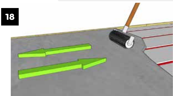
Rol direct de gietmassa door met een prikkerroller
